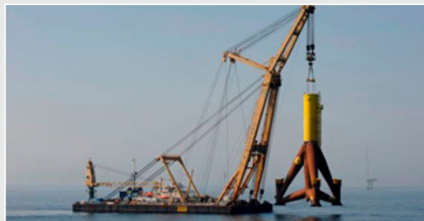
Shearleg crane-barge
